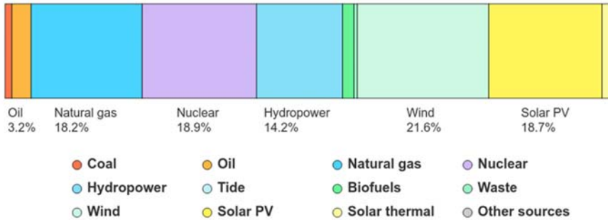
Figure 26. Mix électrique espagnol en 2024
