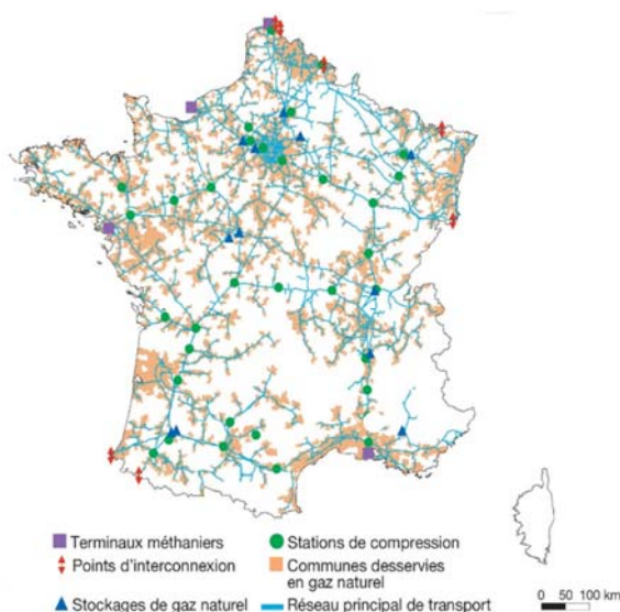
Figure 6. Architecture du réseau gazier français au 31 décembre 2023 3 .
