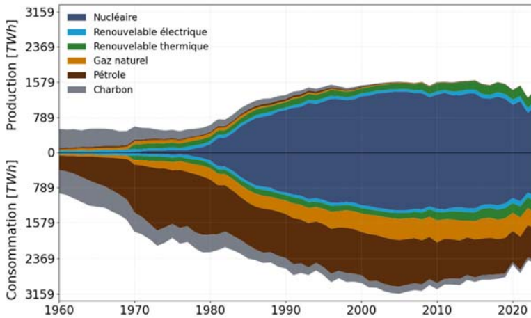
Figure 2. Production et consommation d'énergie primaire en France 1 .
