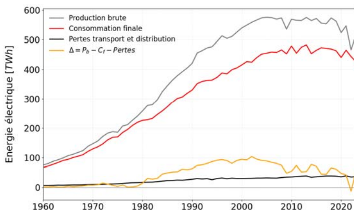
Figure 8. Bilan électrique de la France depuis 1960 2 .
