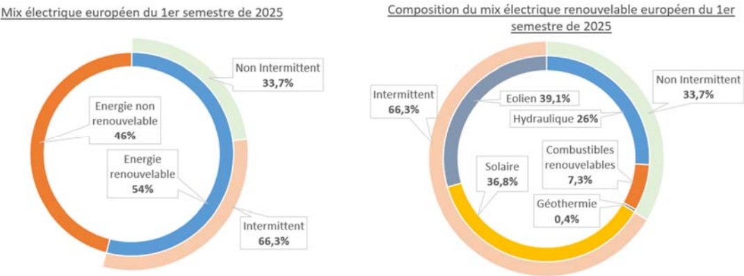
Figure 24. Production finale d’électricité en Europe au 1 er semestre 2025.
