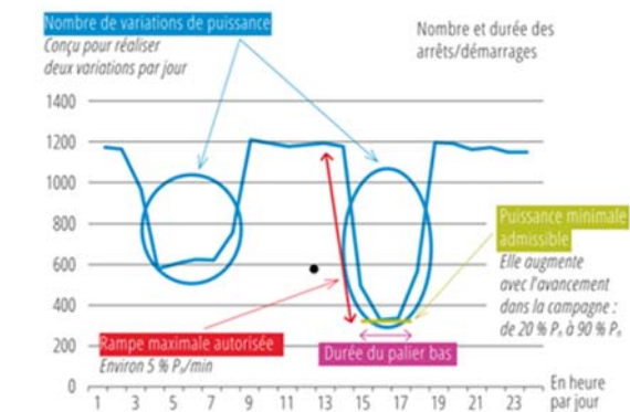
Figure 15. Capacité de suivi de charge d'un réacteur nucléaire (Cattenom 2, 15 août 2014) Crédit : Nicolas Mounier ( https://x.com/nmounier16/status/1655662158783340544 )
