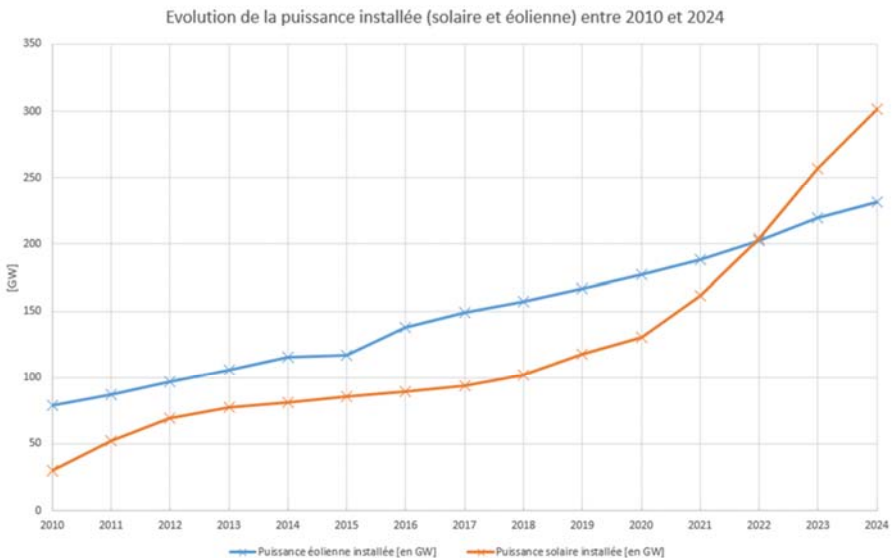
Figure 23. Capacité installée d'énergies solaire et éolienne en Europe 2010 - 2024.
